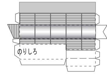
隅棟 4
